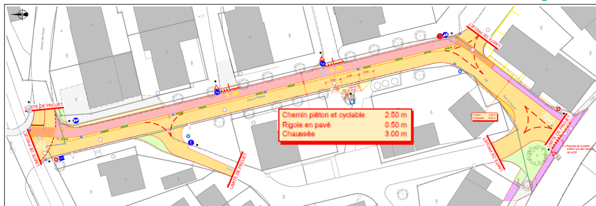
Plan des aménagements et profil de la route (source : plans ATB SA)
